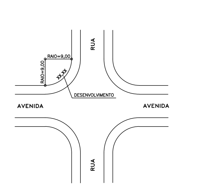
DETALHE DO CRUZAMENTO DAS VIAS (SEM ESCALA)
