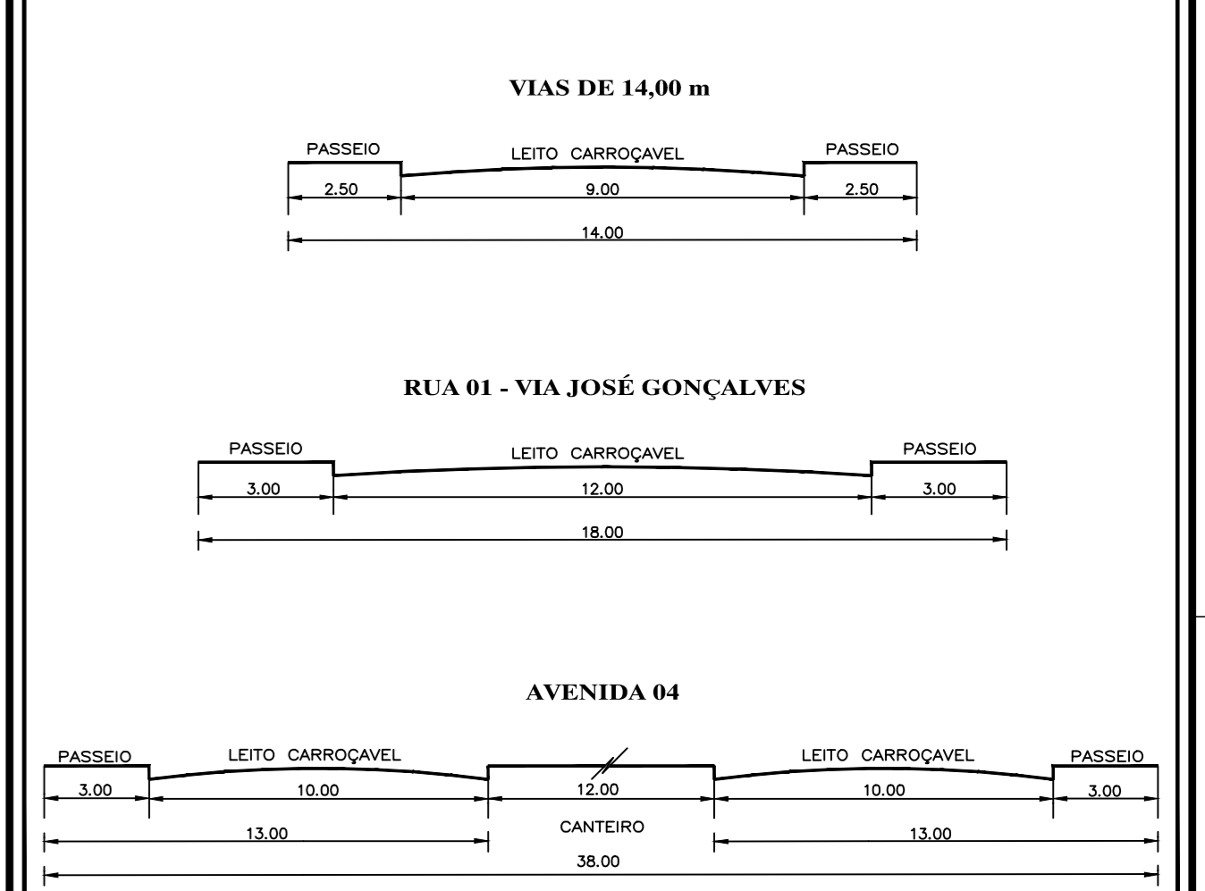
SEÇÃO TRANSVERSAL DAS VIAS (SEM ESCALA)
